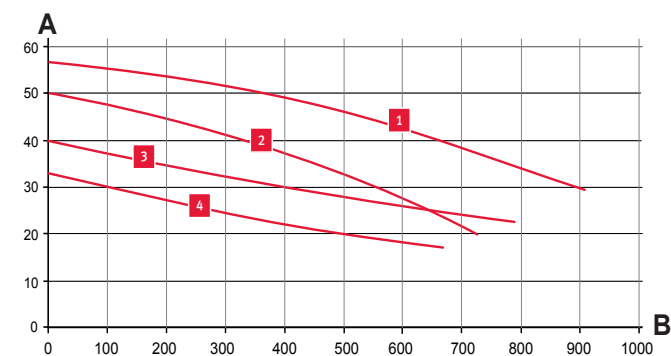
Curva portata/prevalenza disponibile all'impianto: THEMA 3 30 SE.
